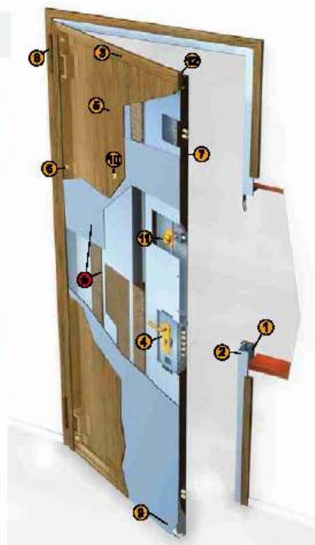
Fire insulation: rock wool Izolacja ognioodporna: wełna mineralna
